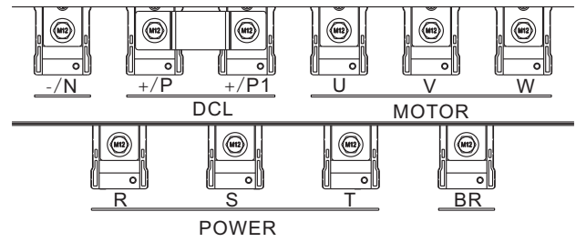
Size J(380V)(280~355kW)
